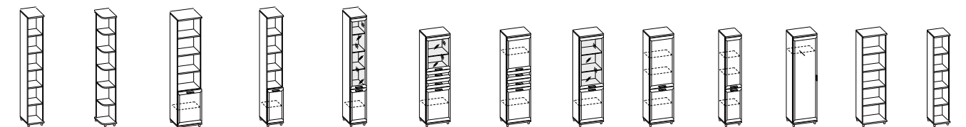
ШК-2851 Шкаф 2264x360x346 ШК-2852 Шкаф 2264x283x346 ШК-2855 Шкаф 2264x540x352 ШК-2856 Шкаф 2264x360x352 ШК-2857 Шкаф 2264x360x352 ШК-2870 Шкаф 1904x540x352 ШК-2872 Шкаф 1904x540x352 ШК-2873 Шкаф 1904x540x352 ШК-2875 Шкаф 1904x540x352 ШК-2876 Шкаф 1904x360x352 ШК-2877 Шкаф 1904x540x352 ШК-2878 Шкаф 1904x540x346 ШК-2879 Шкаф 1904x360x346
